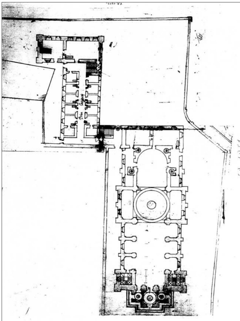
1 pav. Vilniaus Šv. Kazimiero bažnyčios ir jėzuitų profesų namų ansamblio projektas; bažnyčios brėžinys 1604 m (?). Reprodukcija iš autorės asmeninio archyvo
